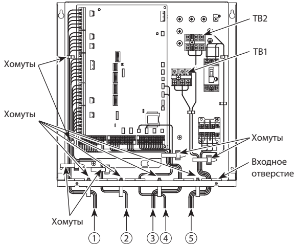
Рис. 4.1.4 Проводка PAC-IF062/063B-E
